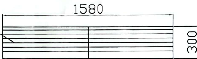
一层栅栏网格放大
